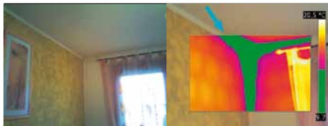
Zone con formazione di muffe
