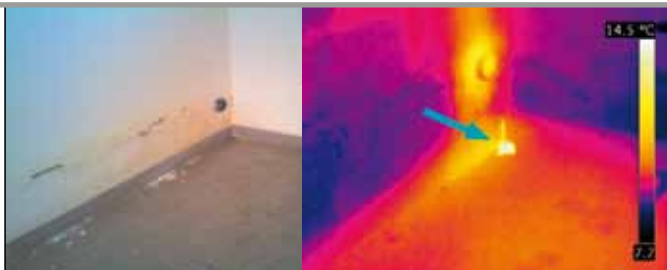
Individuazione della perdita e della relativa umidità di risalita
